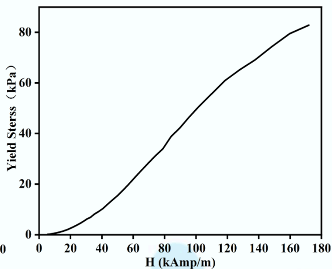
Fig 2: 25°C屈服应力与磁场强度关系
