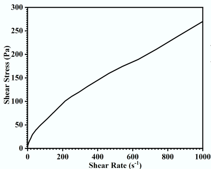
Fig 1: 25°C零磁场下剪切应力与剪切速率关系
