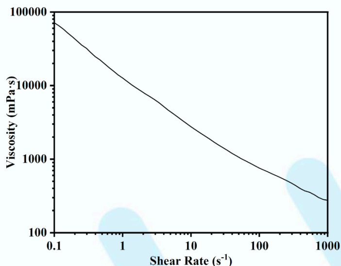
Fig 3: 25°C剪切速率与黏度关系
